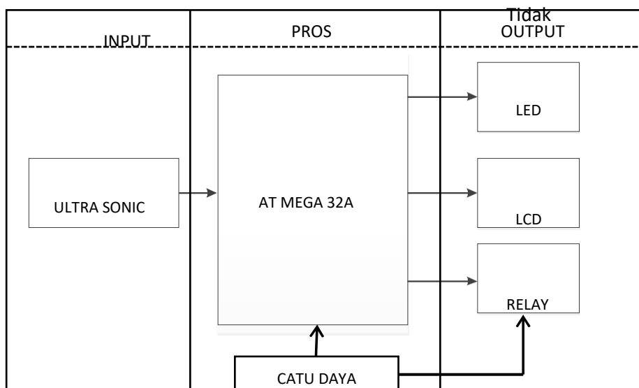
Gambar 4. Blok Diagram Sistem
