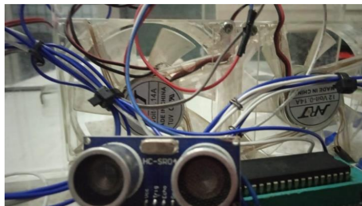
Gambar 6. Rangkaian Sensor Ultrasonik
