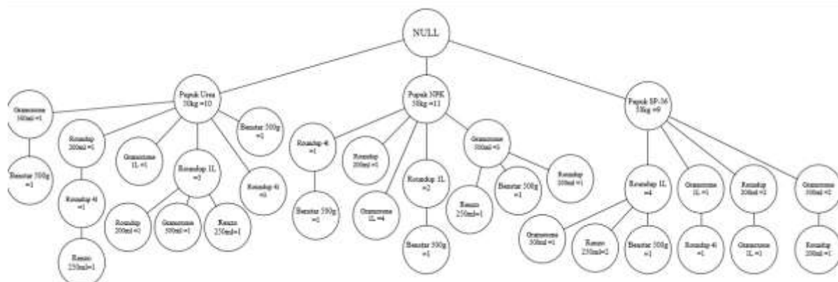
Gambar 2. Hasil Pembentukan akhir FP-tree transaksi T30
