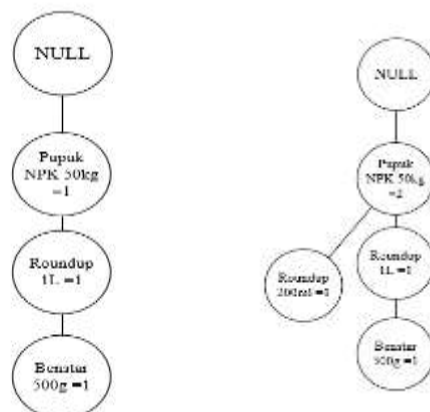
Gambar 1. hasil pembentukan FP-tree T01 dan T02 setelah pembacaan transaksi
