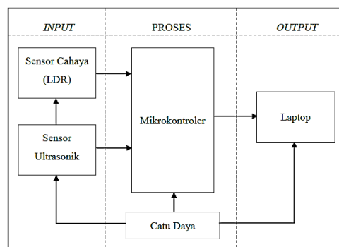
Gambar 6 Blok Diagram Kecerdasan Otomatis dan Peringatan Jarak
