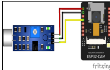
Gambar 11. Rangkaian Sensor Suara
