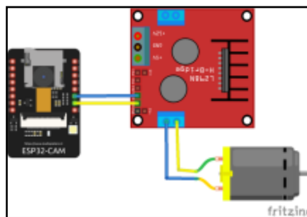
Gambar 10. Rangkaian Motor DC
