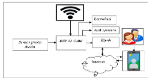
Gambar 4. Arsitektur Pengiriman Data Server-Client
