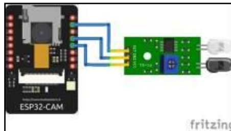
Gambar 9. Rangkaian Sensor Photodioda
