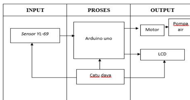
Gambar 2.4 Blok Diagram.
