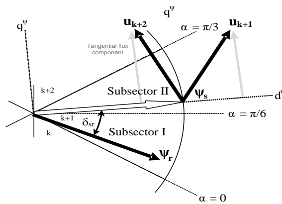
Gambar 1. Efek memilih switching yang berbeda dalam kondisi dinamis
